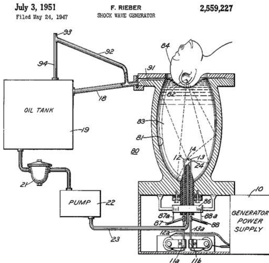
Рис. 1. Перша модель генератора хвиль Ф. Рейбера.
