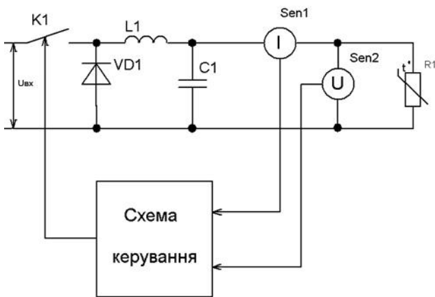
Рис. 2. Спрощена структурна схема ЕХВА.
