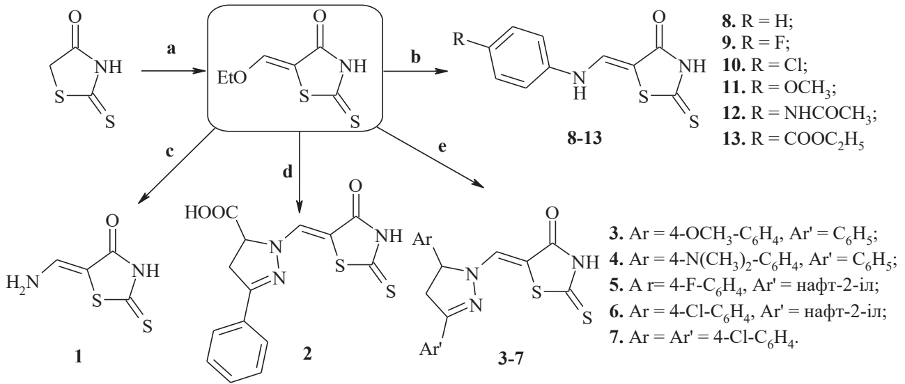
Рис. 1. Синтез похідних 5-амінометилена-2-тіоксотіазолідин-4-ону 1-13 .
