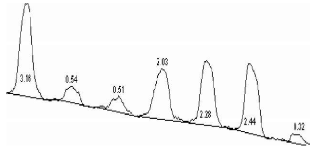
Рис. 11. Фрагмент профільного графіка (для першого рядка плям).
