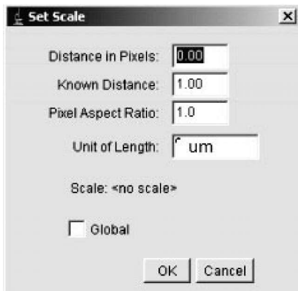
Рис. 3. Вікно шкал.
