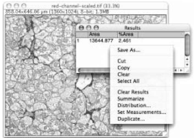
Рис. 15. Вікно результату.
