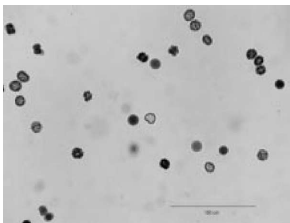
Рис. 2. Вихідне зображення.
