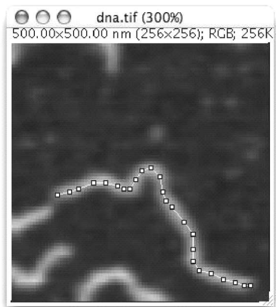
Рис. 8. Вибраний ДНК-контур.
