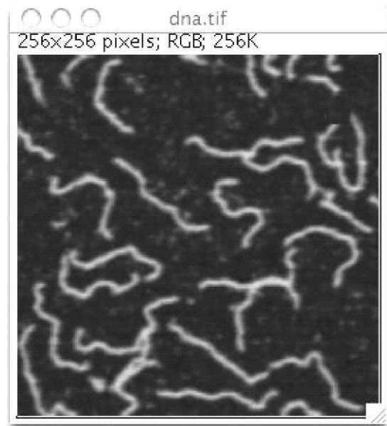
Рис. 6. Зображення фрагмента ДНК, нанесеного на слюду.
