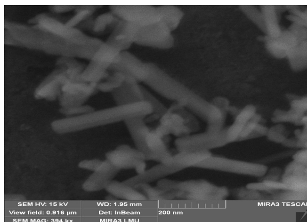
Рис. 2. Микрофотография наночастиц кристаллов стронциевого гидроксилапатита, полученного методом осаждения из нитрата стронция.
