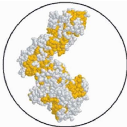
Рис. 1. Гідродинамічний радіус пептидів: інсулін, імуноглобулін G та лізоцим [8].
