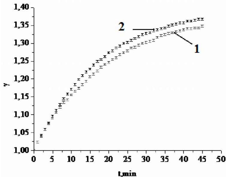
Рис. 1. Часові залежності коефіцієнта відносної зміни температури муцинового гелю (1 - немагнічений гель, 2 - гель, попередньо витриманий в постійному магнітному полі).
